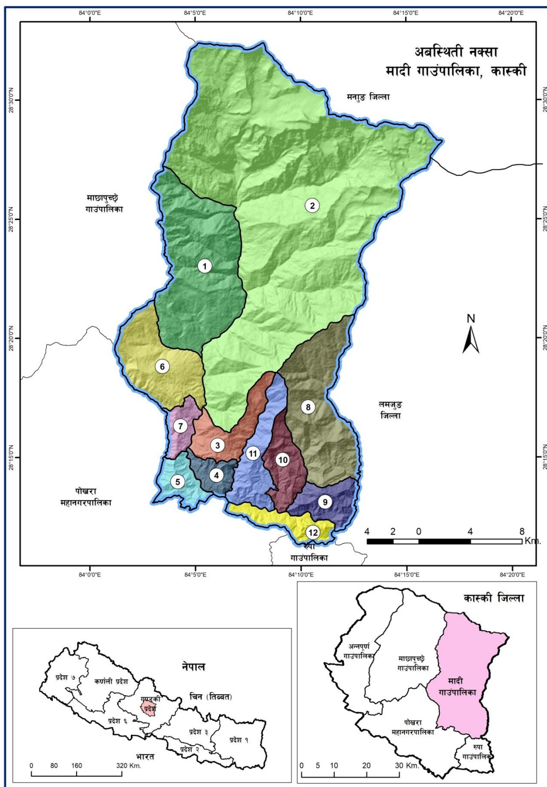
नक्सा २.१: गाउँपालिकाको अबस्थिति नक्सा
